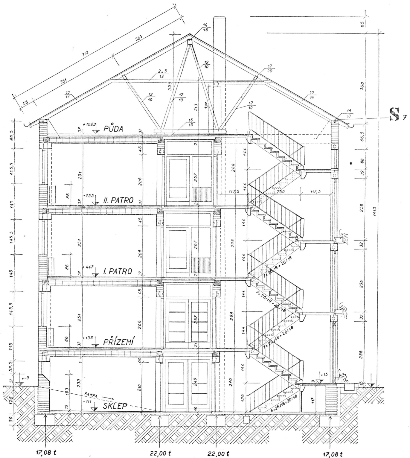
ŘEZ A-A
