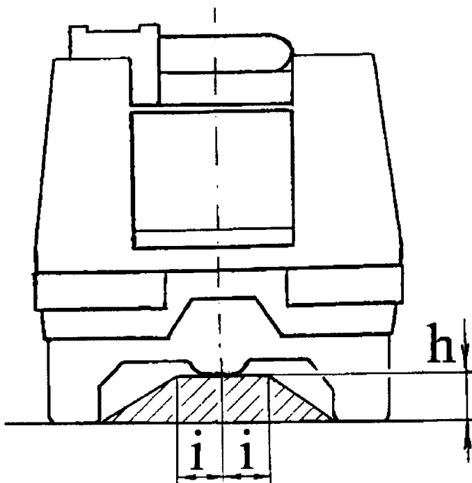
Obr. 4 Světlá výška nad zemí pod nápravami h (hodnota „ i “ je vždy 0,3 m)
