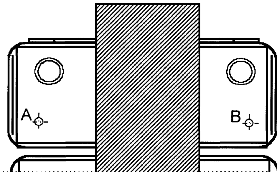
Obr. 7c Antény komunikačních prostředků umístěny v příčné ose na střeše kabiny osádky s jednou řadou sedadel, „A“: anténa pro 160 MHz, „B“: anténa pro 380 MHz
